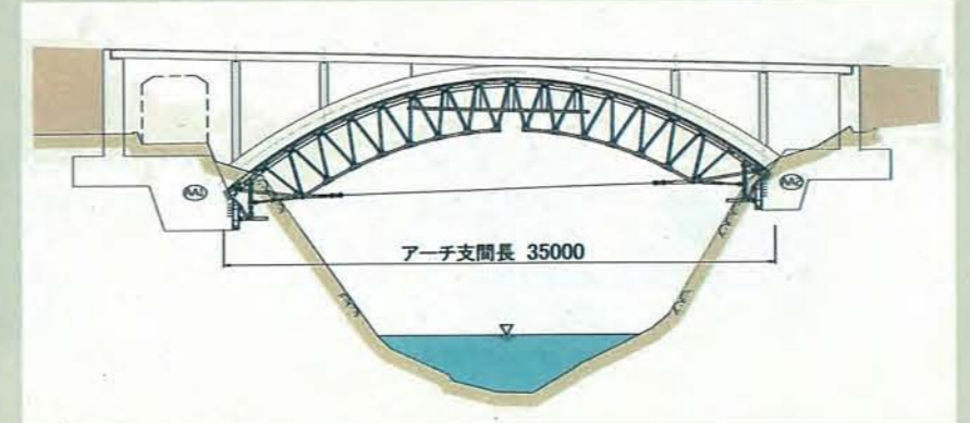
■図2—鋼製アーチセトル工法による架設
